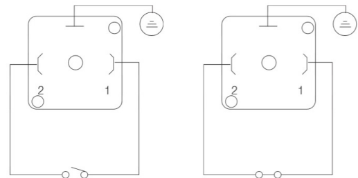
TWR-5101, -5201
